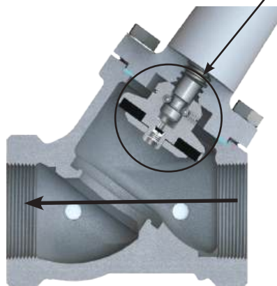
ME825IBC-16 Patentada en EE.UU. y Canadá
