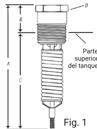
Dimensiones (aprox.) - vea la Fig. 1
