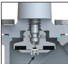
Función de no retroceso integrada (IBC)
