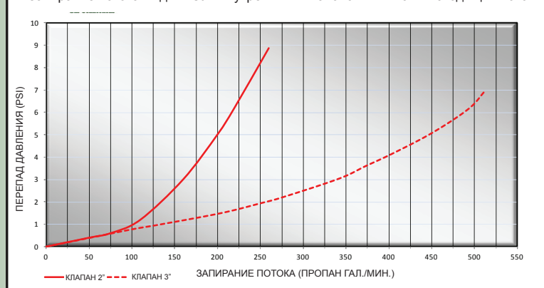
Запирание потока жидких СУГ внутренними клапанами 2" и 3" -нисходящий поток
